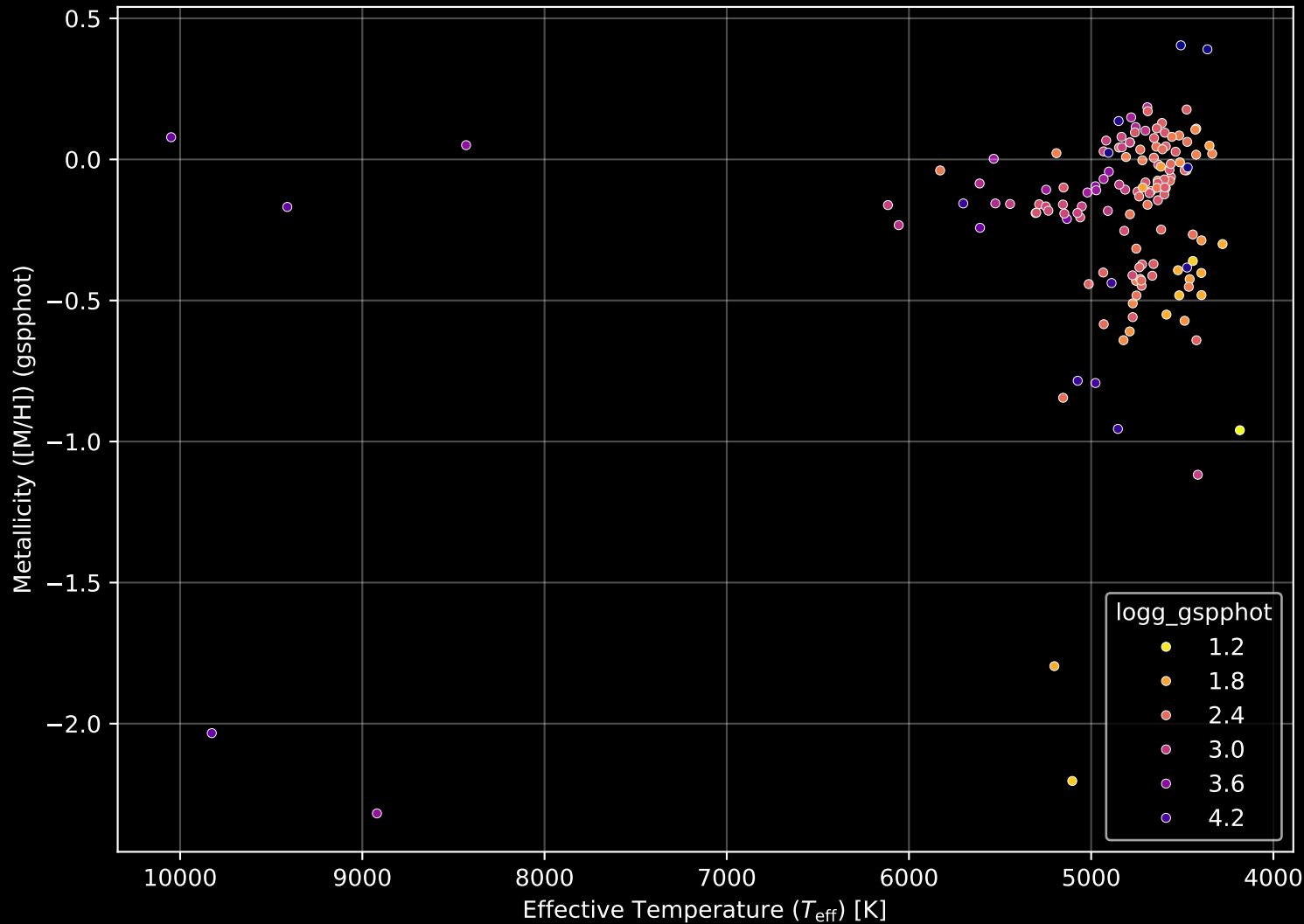
APOGEE DR17 Field: [340-12] Stellar Population Parameters (n= 144)
